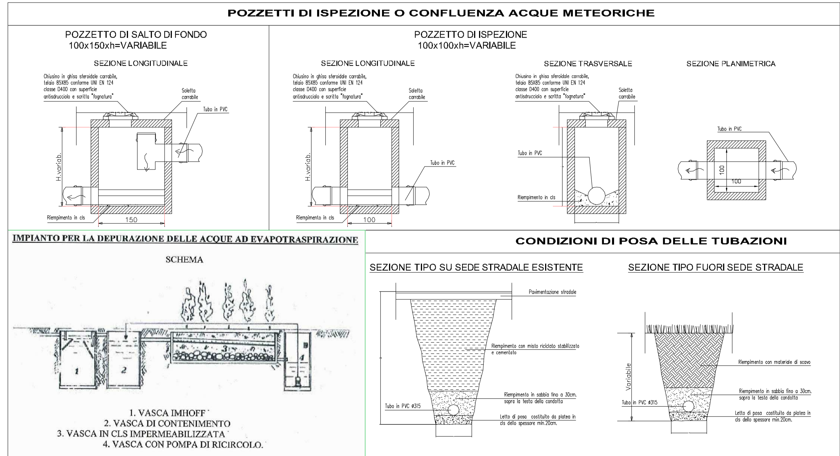
FOGNATURE - scala 1:2.000
